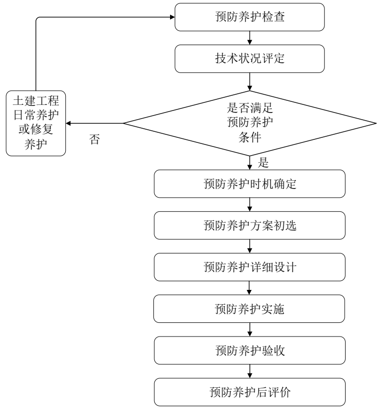
图 1 隧道土建工程预防养护常规工作流程
